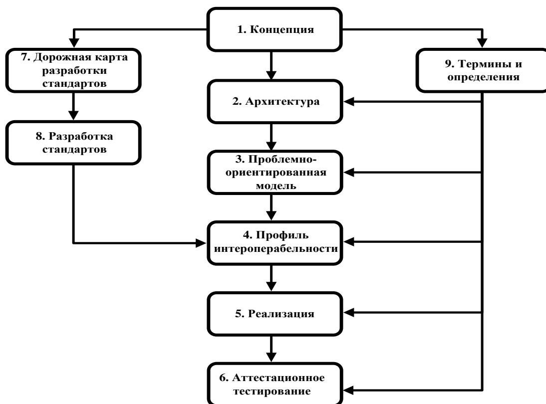
Рисунок 1 – Методика обеспечения интероперабельности грид-вычислений и облачных вычислений.
