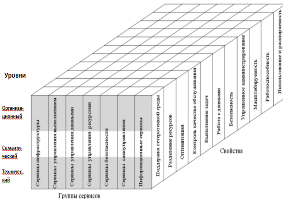
Рисунок 2 - Модель интероперабельности грид-вычислений
